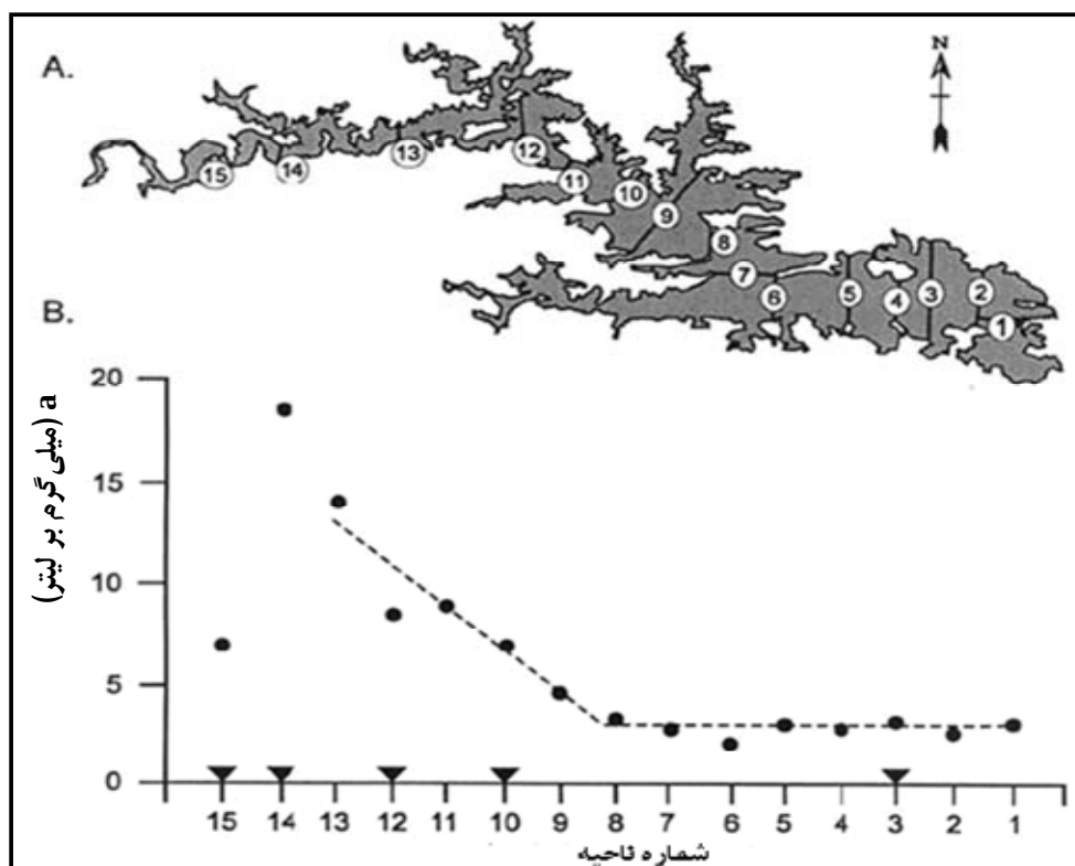
شکل ۷-۲- ناحیه بندی طولی دریاچه دی گری در آمریکا به منظور پایش کیفی- همان گونه که از میانگین نتایج هر مقطع پیداست دریاچه به پنج ناحیه تقسیم و ایستگاه های ۳، ۱۰، ۱۲، ۱۴ و ۱۵ برای تعیین روند تغییرات طولی انتخاب می شوند [۲]
