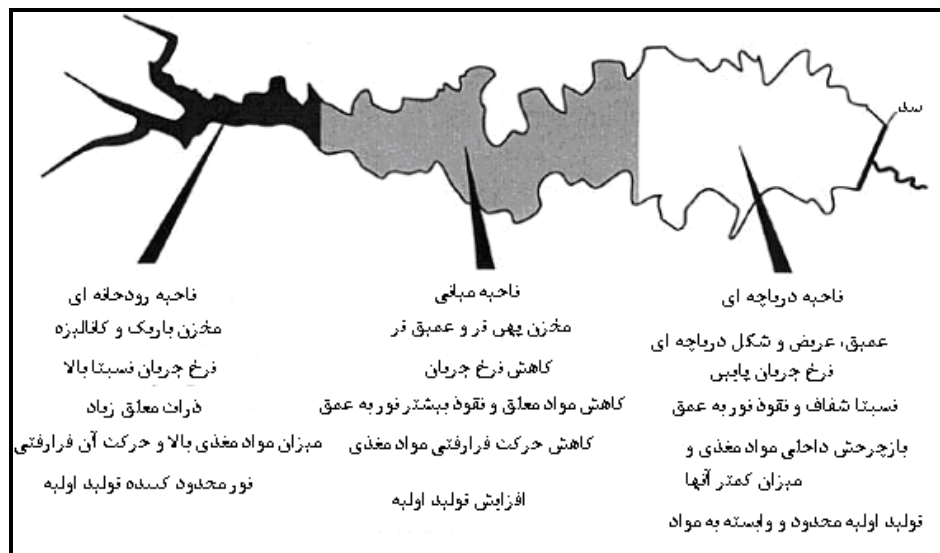
شکل ۷-۱- ناحیه بندی طولی شرایط کیفیت آب در مخازن سدهای رودخانه‌ای
