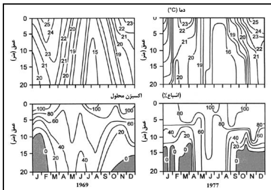
شکل ۴-۷- منحنی‌های هم‌دما و هم غلظت پارامترهای کیفی نسبت به عمق
